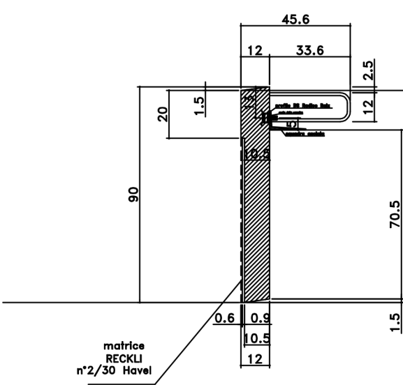
SEZIONE TIPO SCALA 1:10
