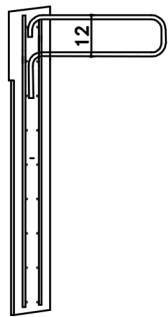
SEZIONE TIPO SCALA 1:10
