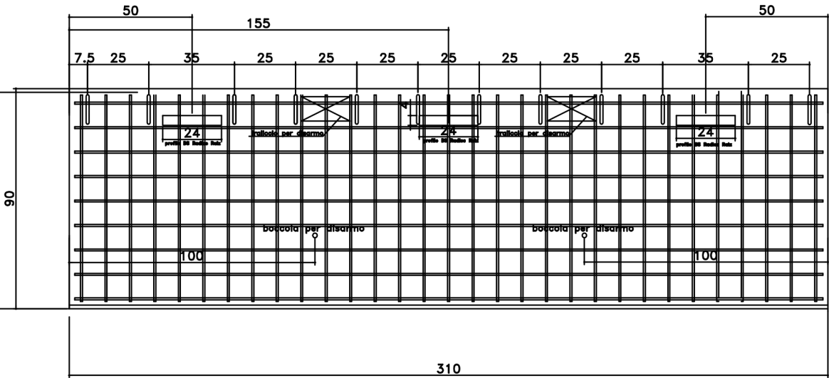
PROSPETTO ARMATURA SCALA 1:10
